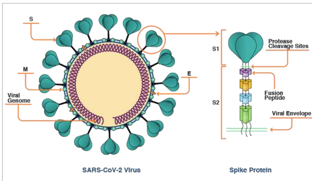
Zgradba S-proteina
